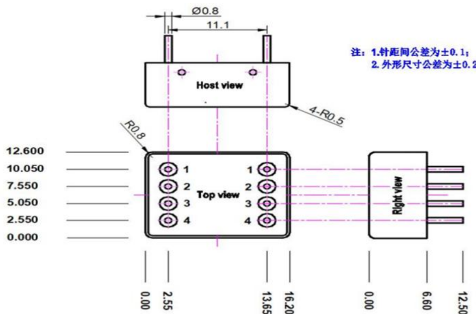
模块尺寸图
