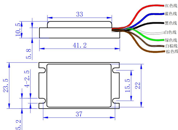
i5外形示意图
